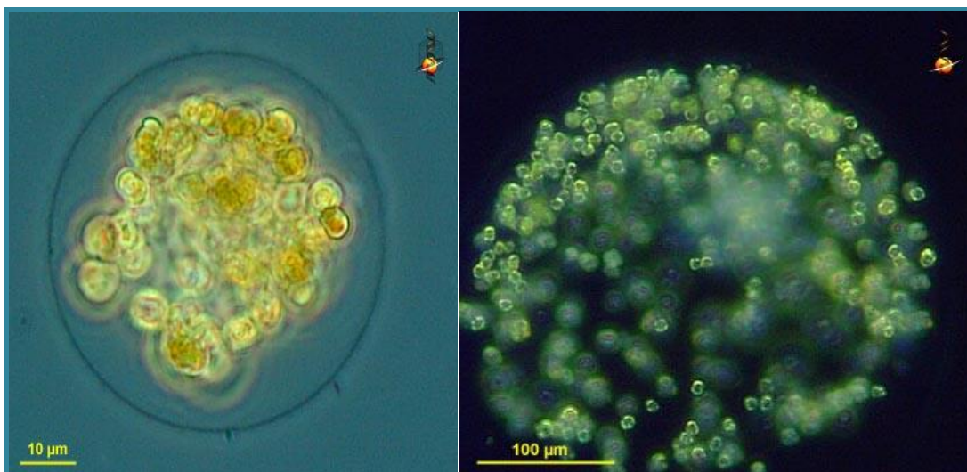
Cellules de Phaeocystis formant des colonies gélatineuses lorsque les nutriments sont présents en abondance. ©Bob Andersen and D. J. Patterson – Courtesy of NCMA
