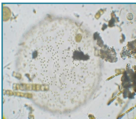
Image des cellules Phaeocystis au microscope Source: PAE Ugent
